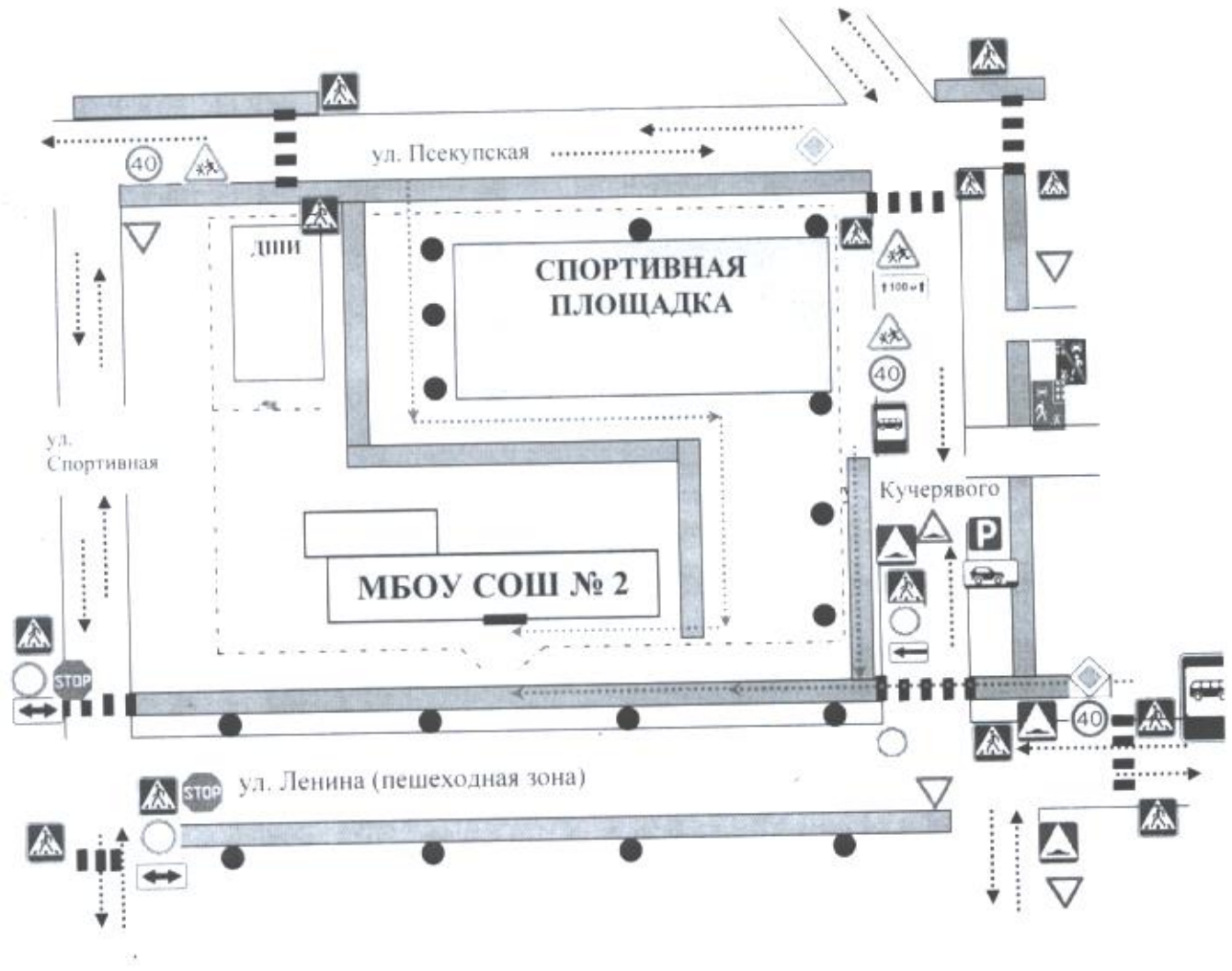
Схема организации дорожного движения в непосредственной близости от МБОУ СОШ №2 с размещением соответствующих технических средств, маршруты движения детей и расположение парковочных мест (объект № 1)
